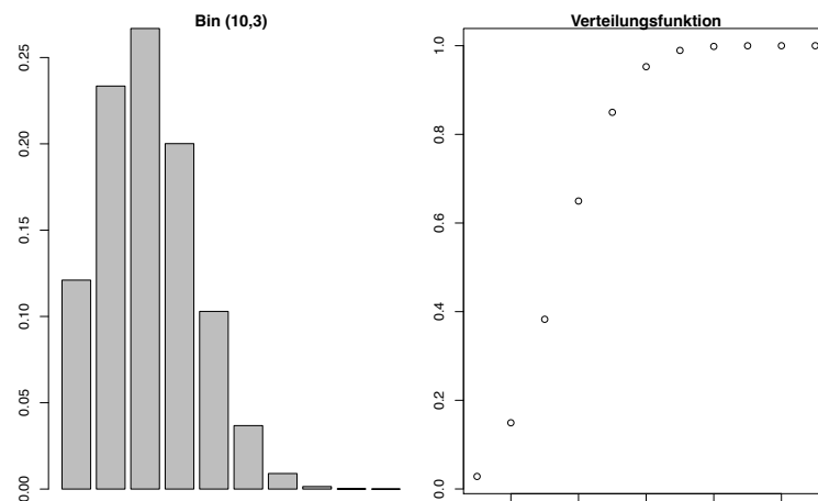
Abbildung 2.1: Verteilungsgewichte und Verteilungsfunktion von B(10, 0.3) .
